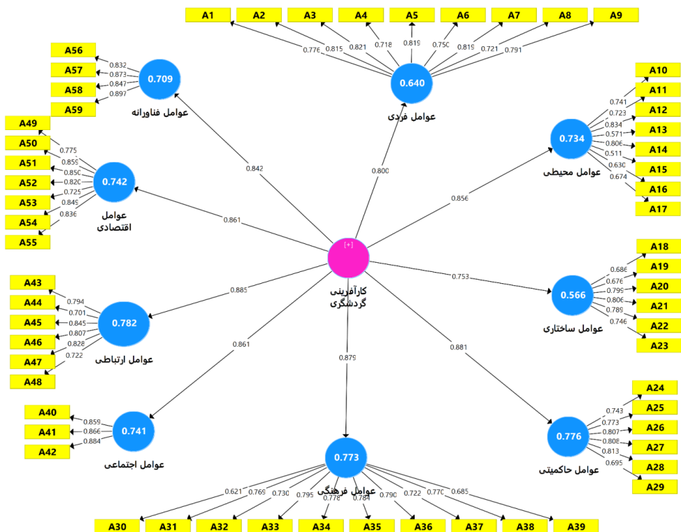
شکل ۱- ضرایب مسیر
